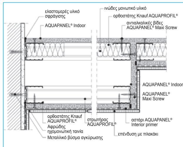
W386-VA1 Σύνδεση τοιχοποιιών διαφορετικού πάχους
